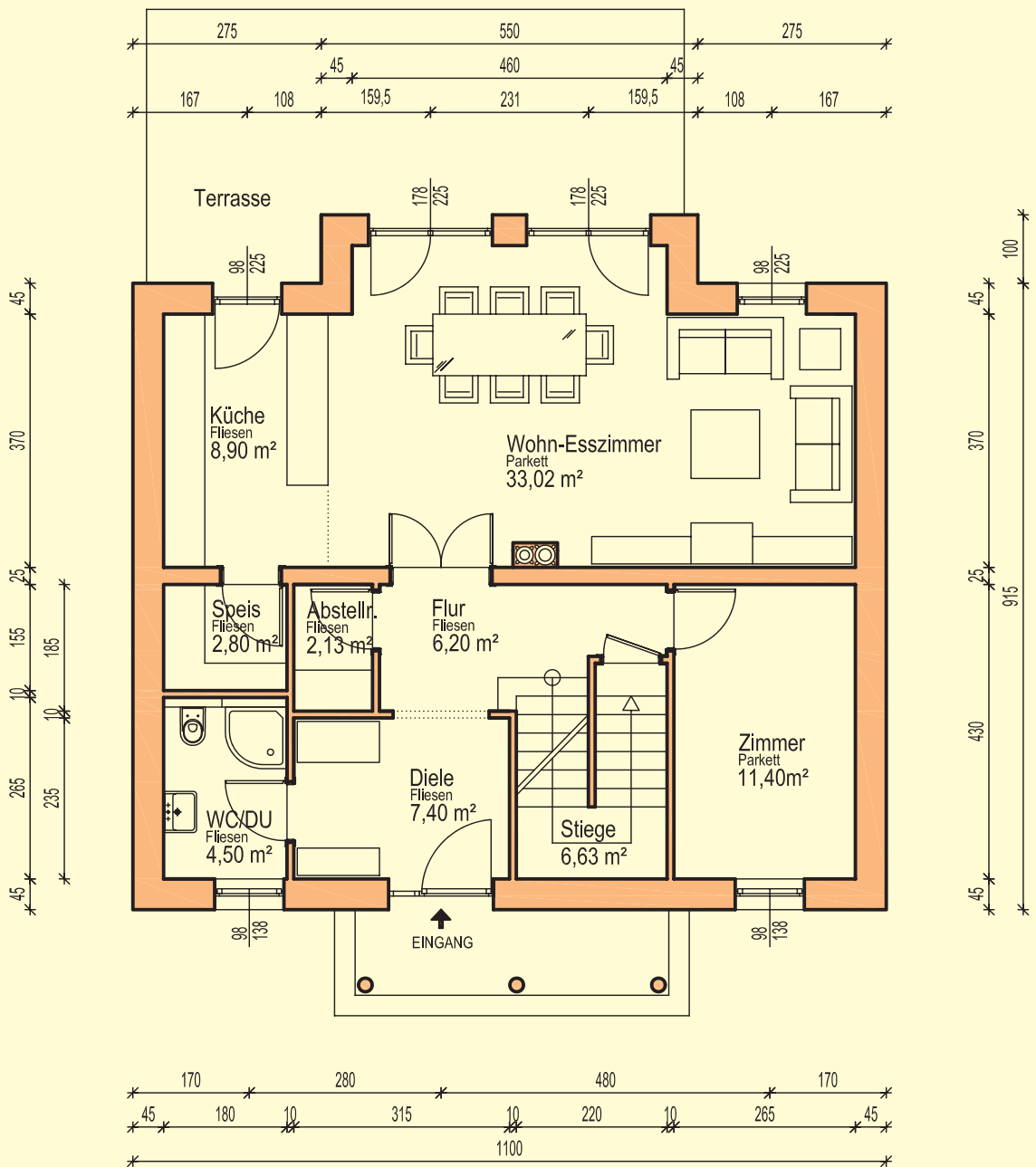
ERDGESCHOSS MASSSTAB = 1:100
