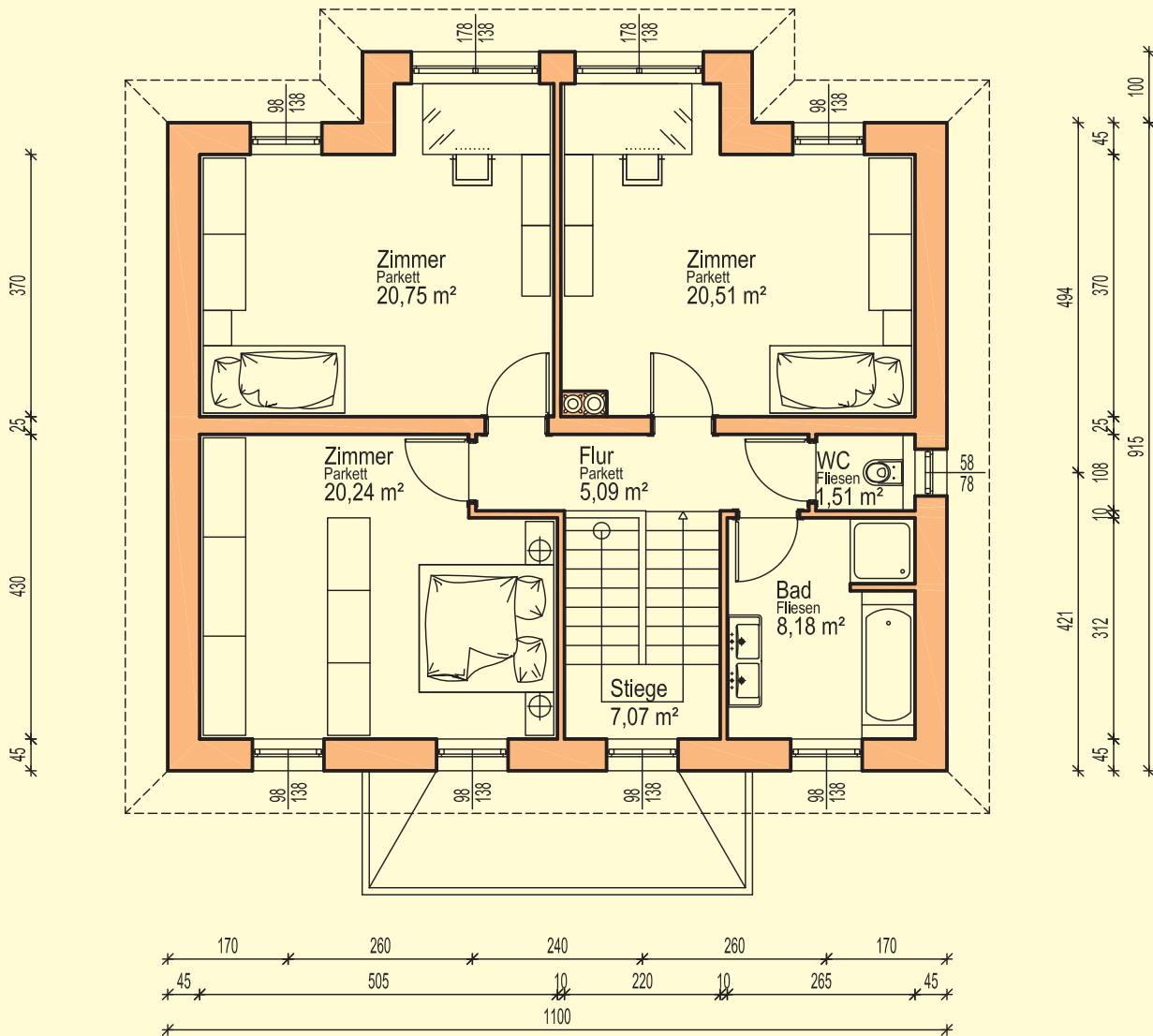
OBERGESCHOSS MASSSTAB = 1:100
